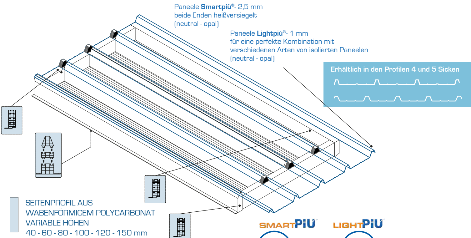
VERSTÄRKTE Ausführung
